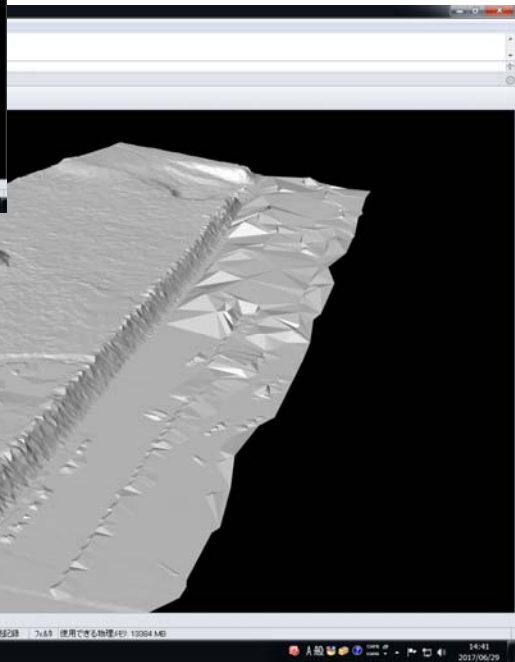
点群データから地形モデル作成 (TIN)
