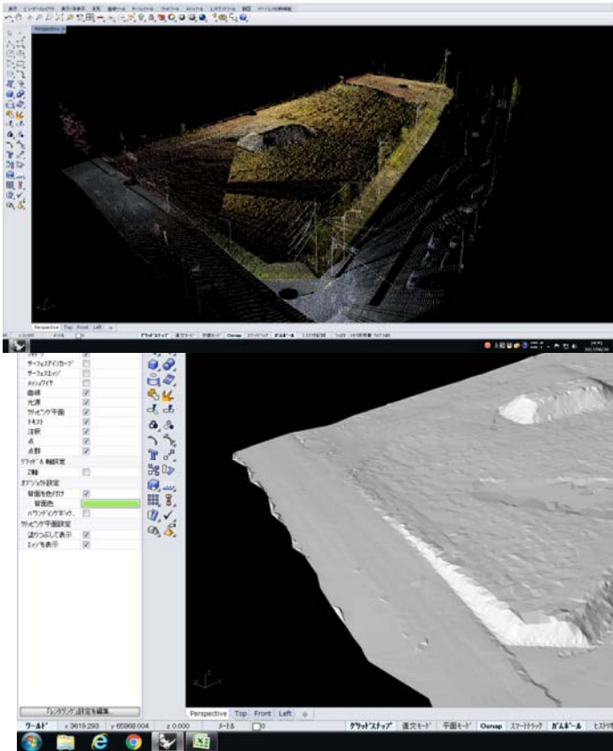
点群データから地形モデル作成 (TIN)
