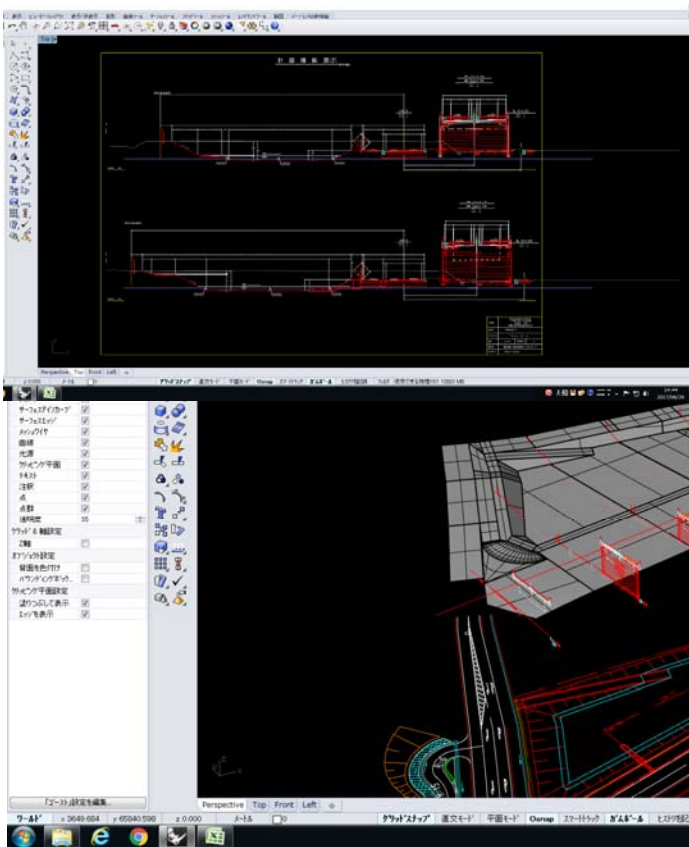
2次元設計図より3次元モデル作成
